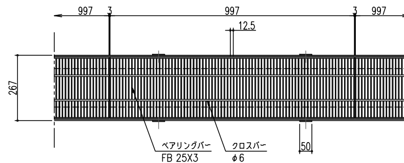
平面詳細図 S=1/10
