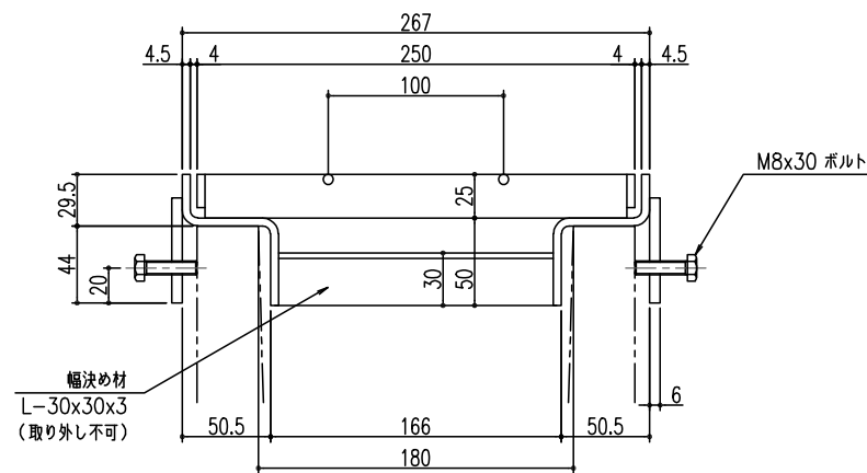
断面詳細図 S=1/3
