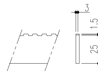
ベアリングバー 詳細図
