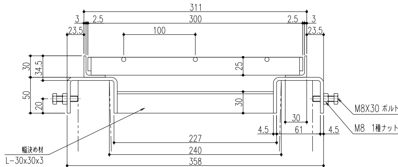
断面詳細図 S=1/3
