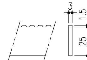
ベアリングバー 詳細図
