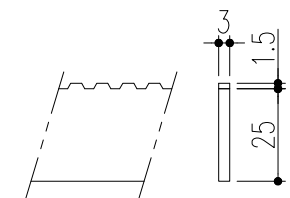
ベアリングバー 詳細図
