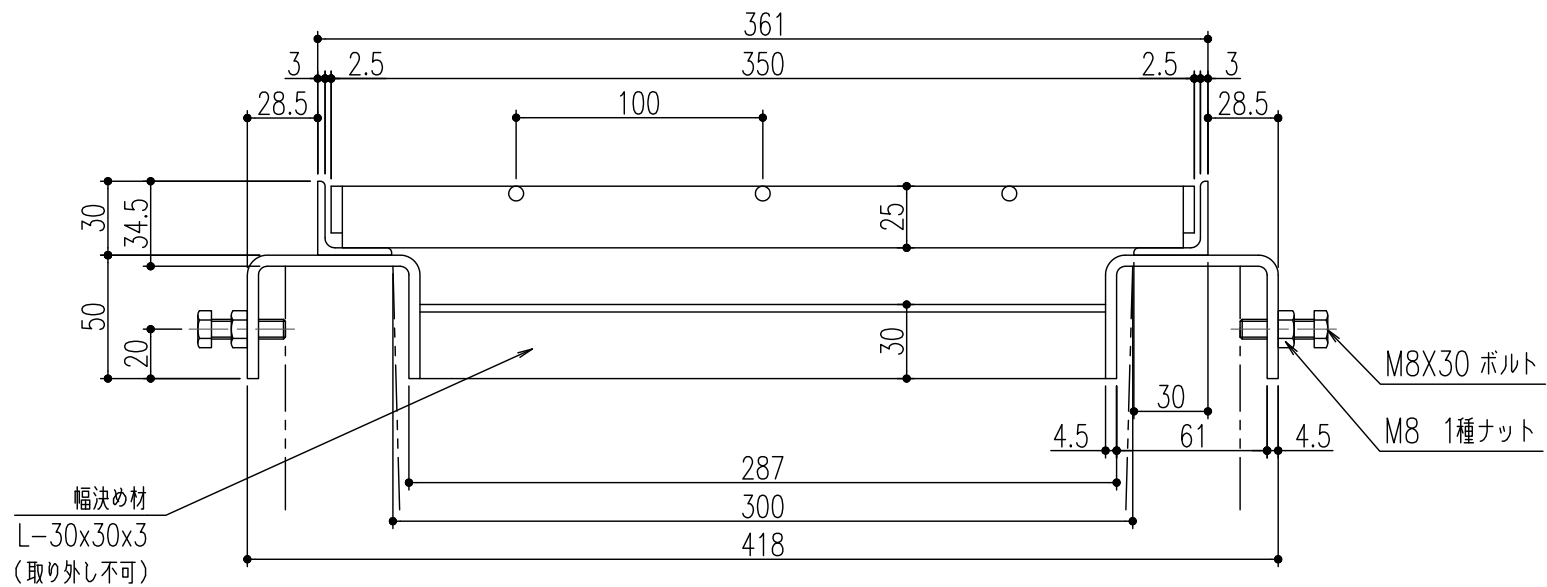
断面詳細図 S=1/3
