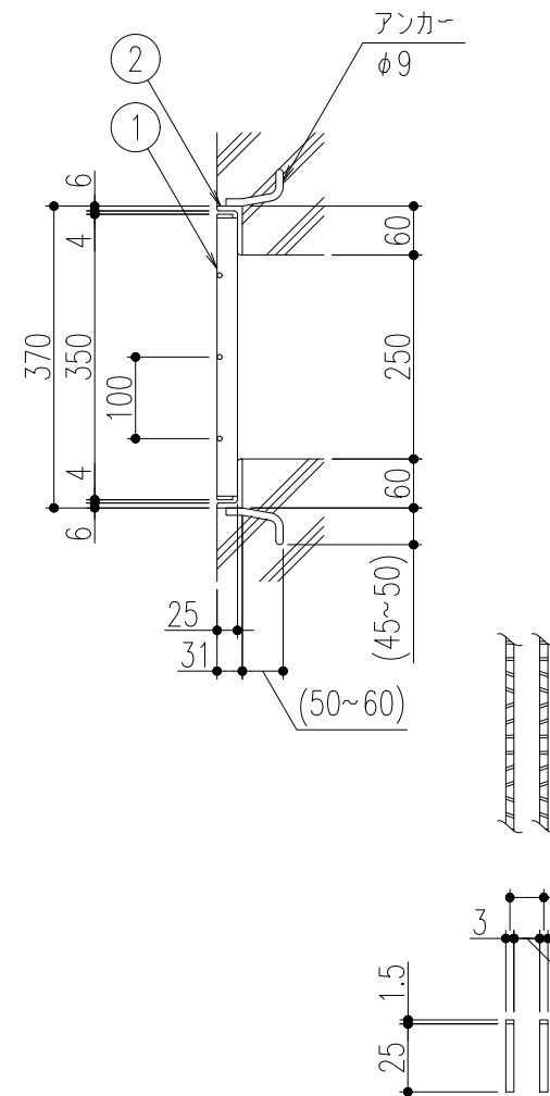
ベアリングバー 詳細図
