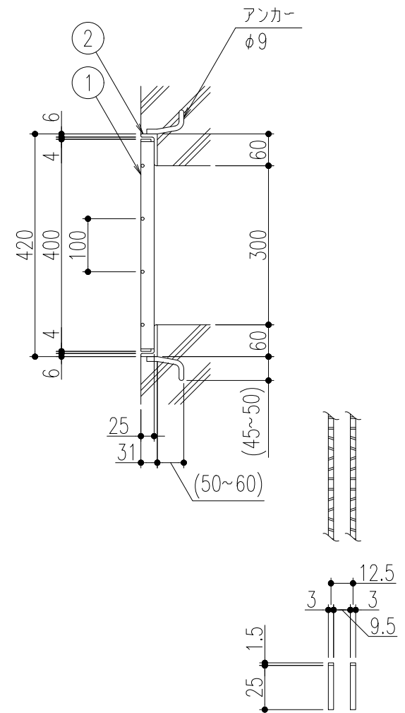
ベアリングバー 詳細図
