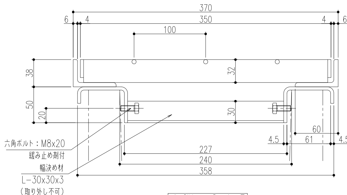
断面詳細図 S=1/3
