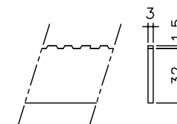
ベアリングバー詳細図
