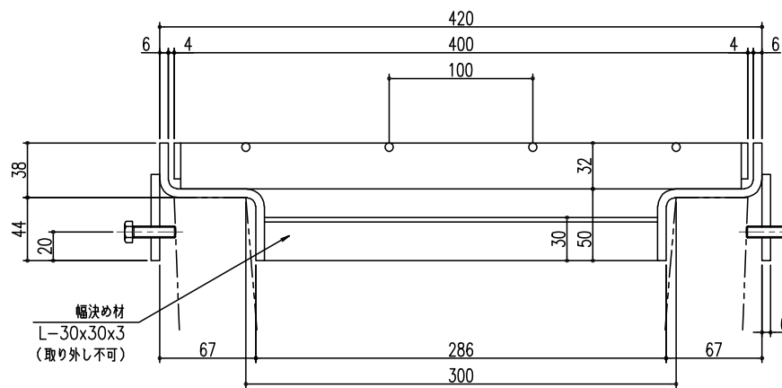
断面詳細図 S=1/3
