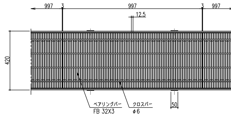
平面詳細図 S=1/10
