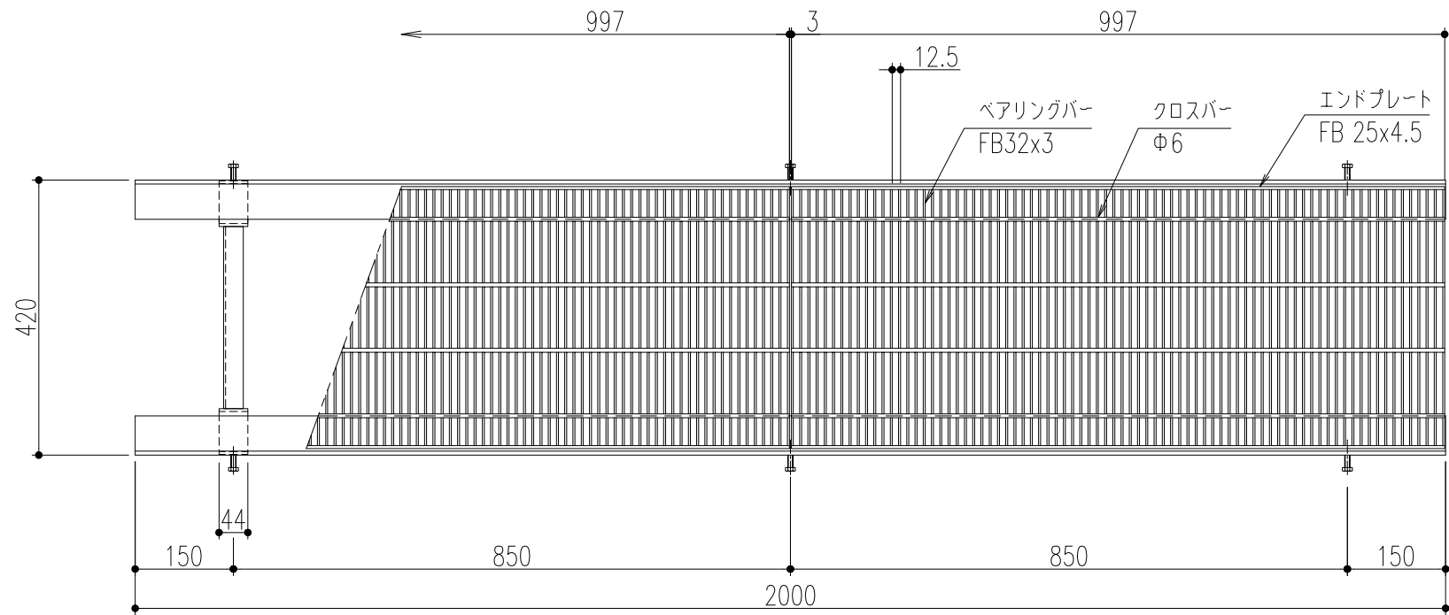
平面詳細図 S=1/10
