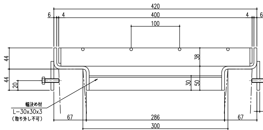
断面詳細図 S=1/3
