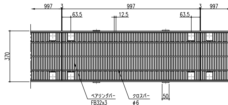
平面詳細図 S= 1/10
