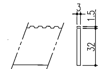
ベアリングバー 詳細図
