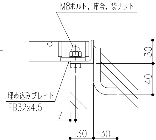
ボルト固定 詳細図
