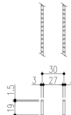
ベアリングバー 詳細図
