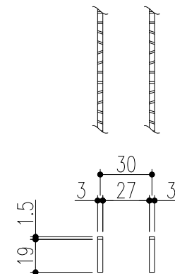
ベアリングバー 詳細図
