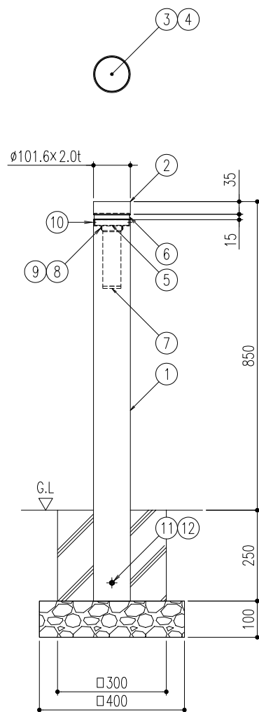
埋込式
