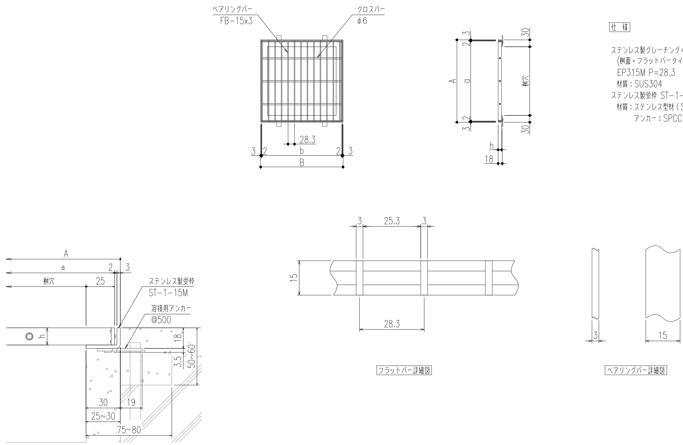
断面詳細図
