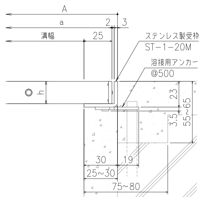
断面詳細図
