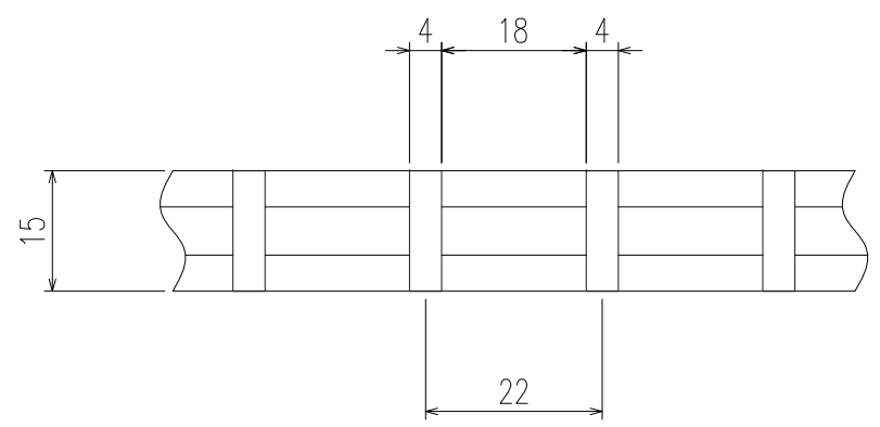
フラットバー詳細図
