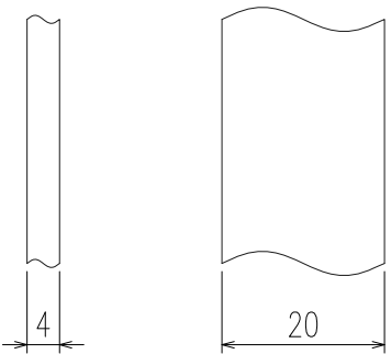
ベアリングバー詳細図
