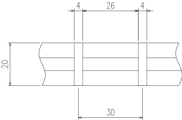
フラットバー詳細図
