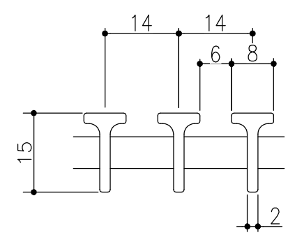
Tバーの断面詳細図
