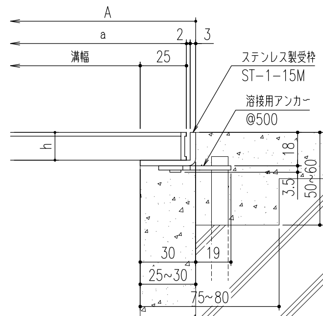
断面詳細図
