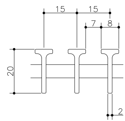
Tバー断面詳細図
