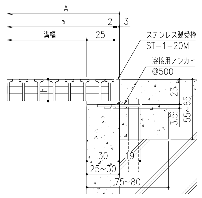
断面詳細図
