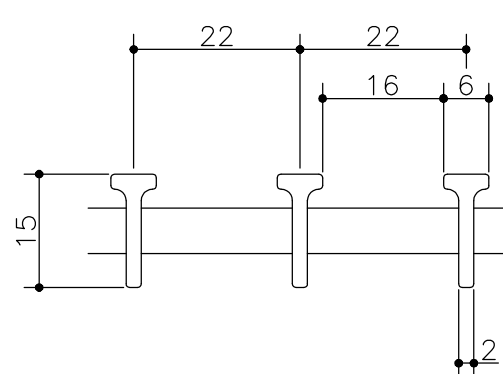
Tバー断面詳細図
