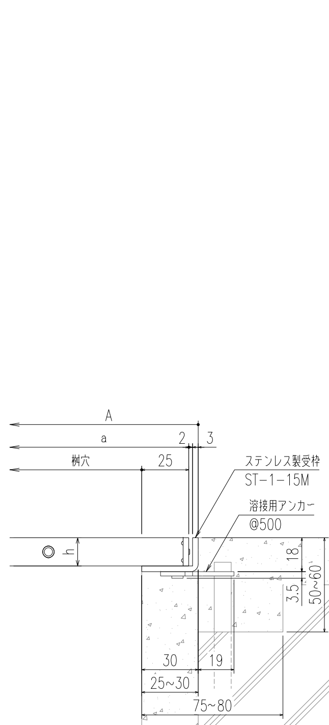
断面詳細図
