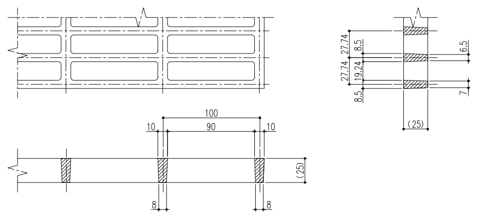
詳細図 S=1/2
