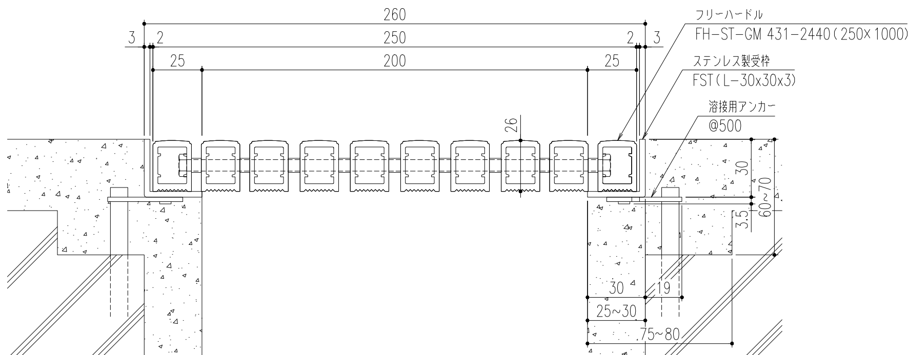
断面詳細図 S=1/2
