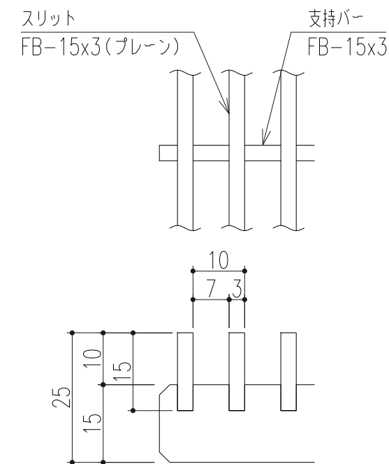
部材詳細図
