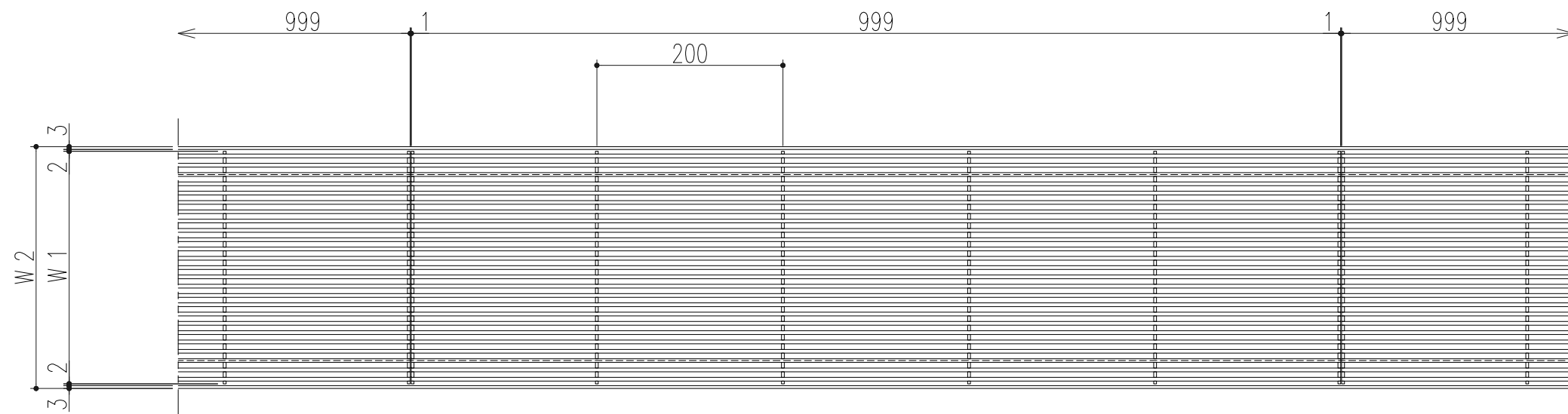
平面詳細図
