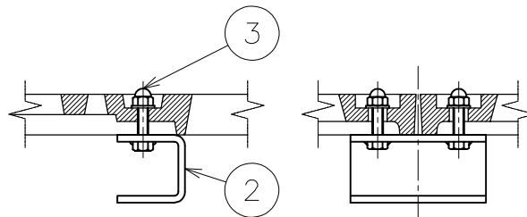
固定部断面 S=1/5
