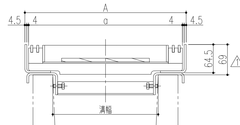
蓋枠納まり断面図 (S=1/5)
