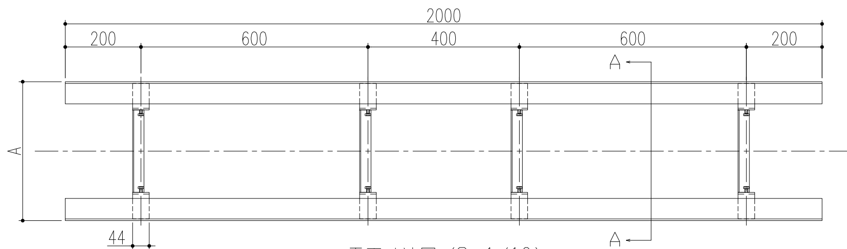
平面寸法図 (S=1/10)
