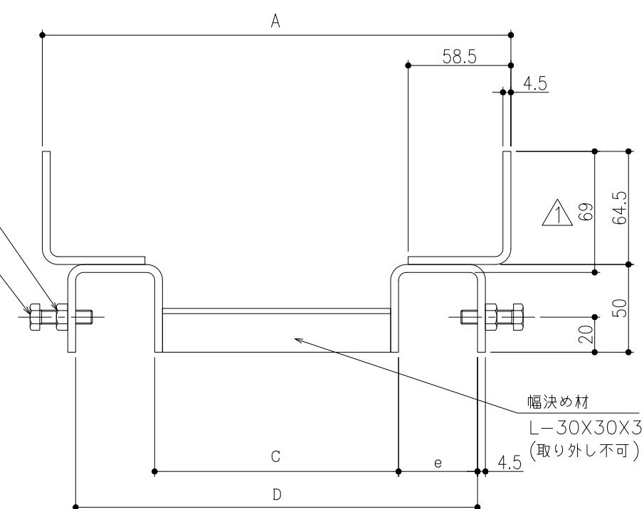
矢視 A-A 断面詳細図 S = 1 / 3
