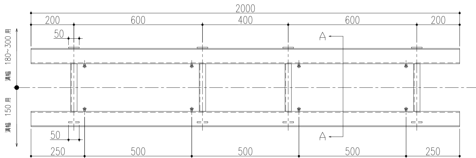
平面寸法図 (S=1/10)
