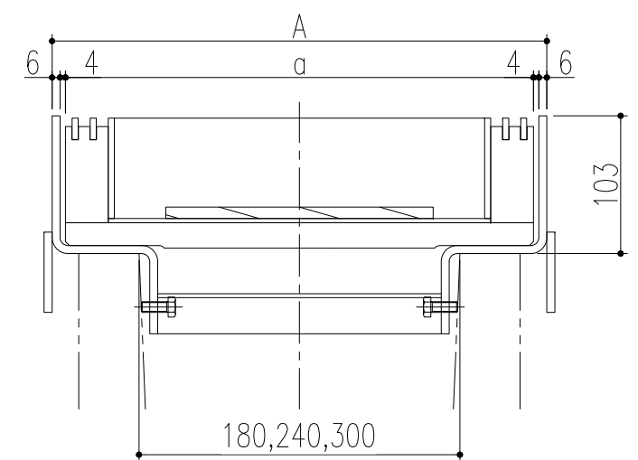
蓋枠納まり断面図 (S=1/5)
