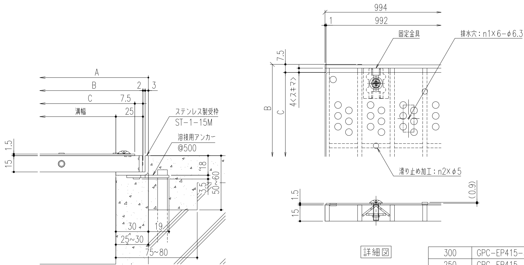
断面詳細図
