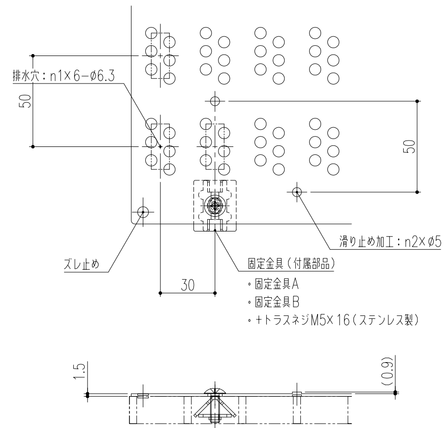
詳細図
