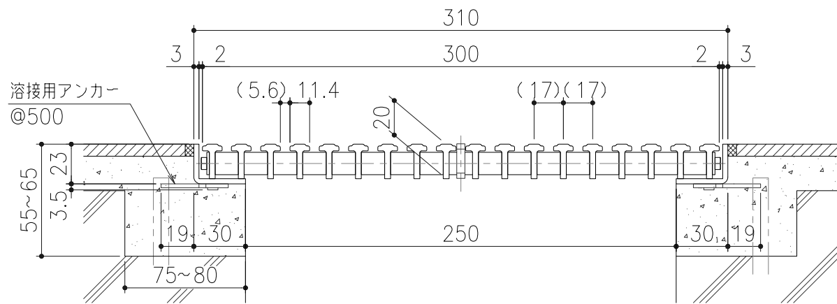
断面詳細図 S=1：3
