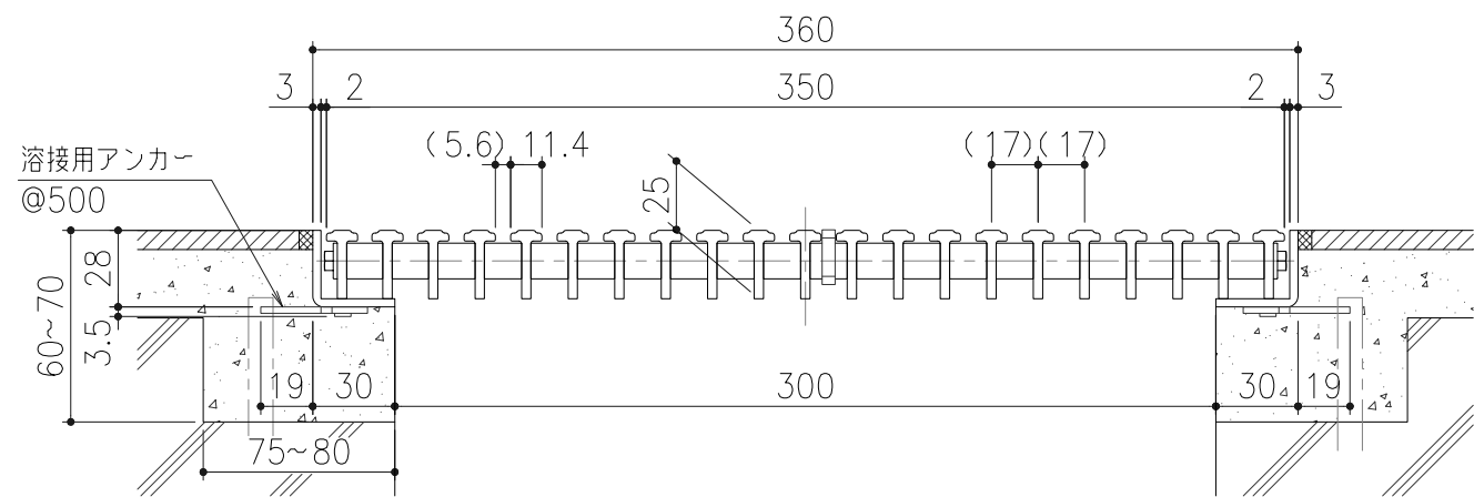
断面詳細図 S=1:3
