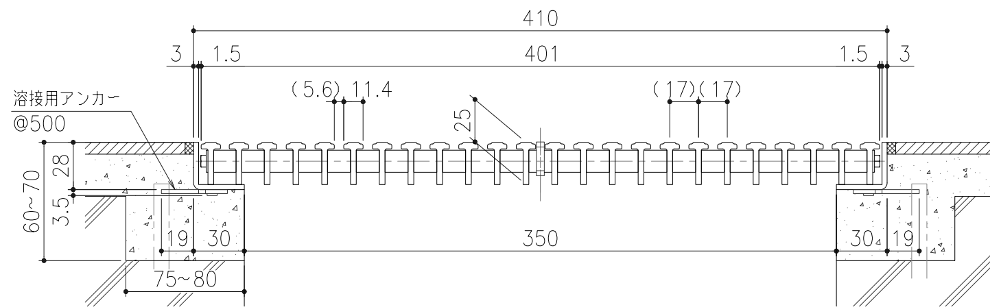
断面詳細図 S=1:3
