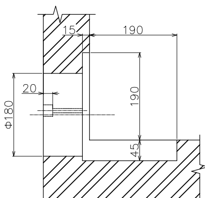
Y-Y断面
