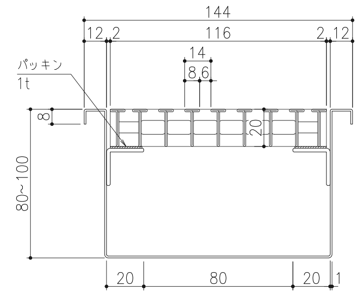
断面詳細図 S=1/2
