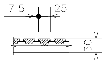
細目断面 S=1/5
