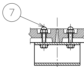
固定部断面 S=1/5
