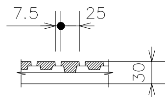
細目断面 S=1/5
