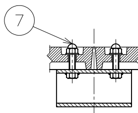
固定部断面 S=1/5
