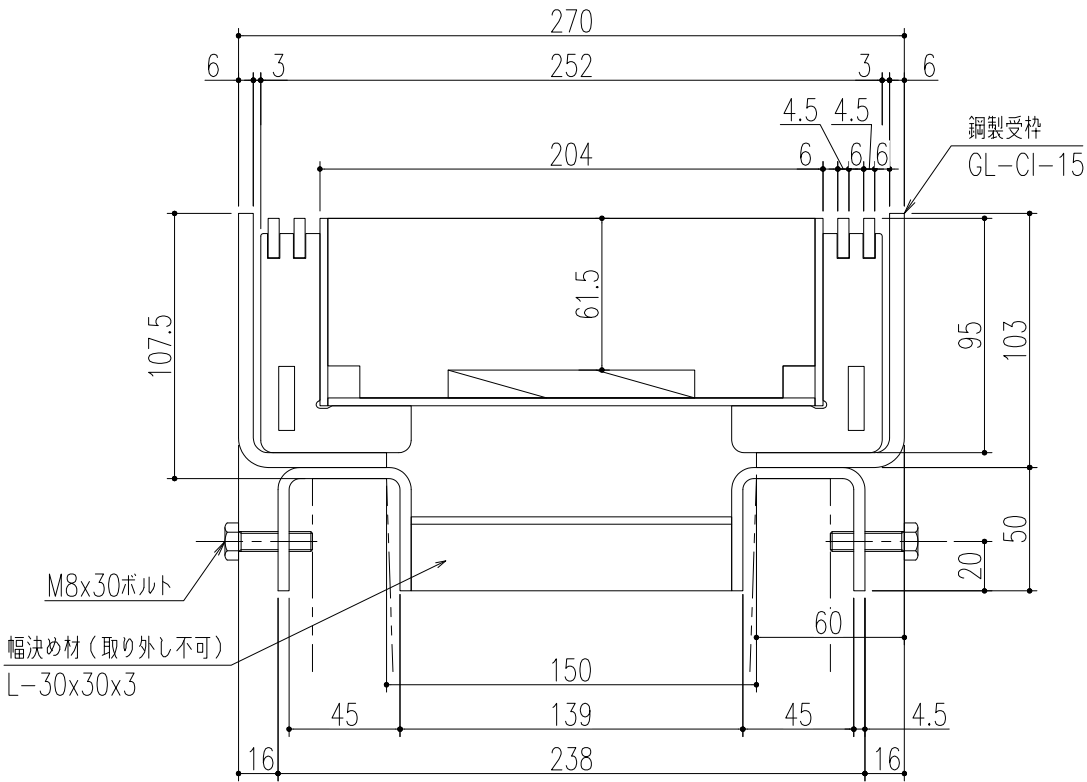
断面詳細図 S=1/3
