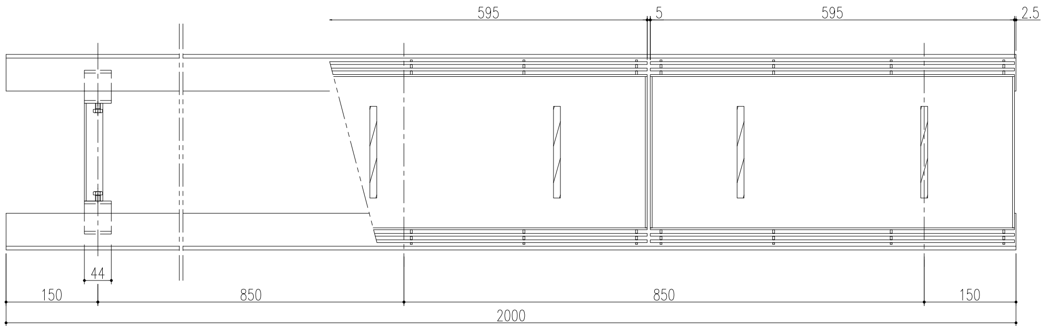
平面詳細図 S=1/6
