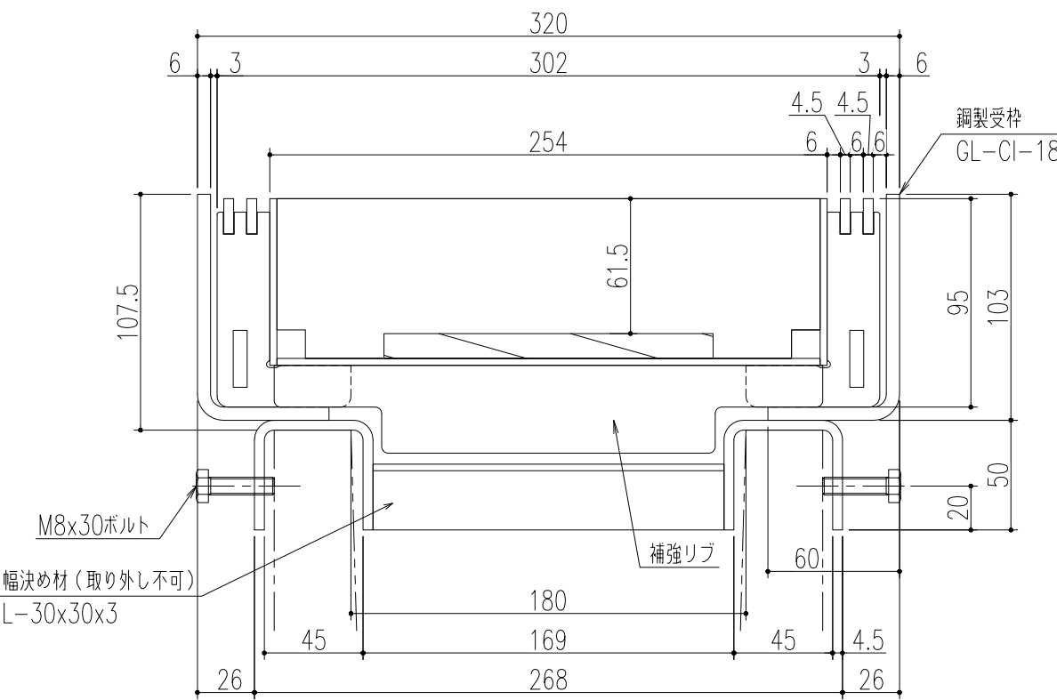
断面詳細図 S=1/3
