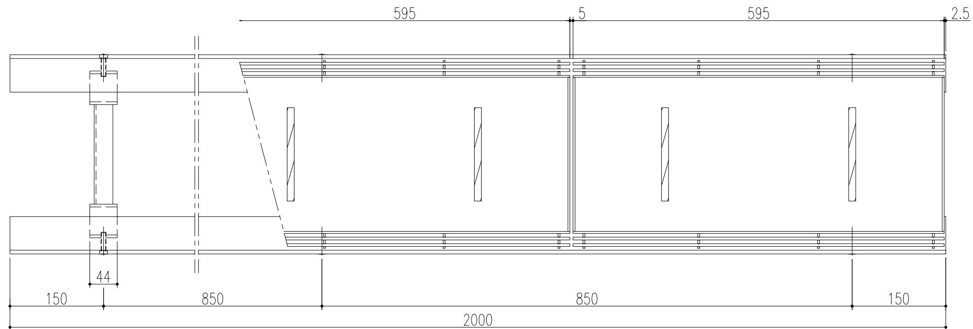
平面詳細図 S=1/6
