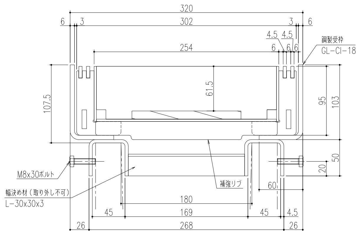
断面詳細図 S=1/3
