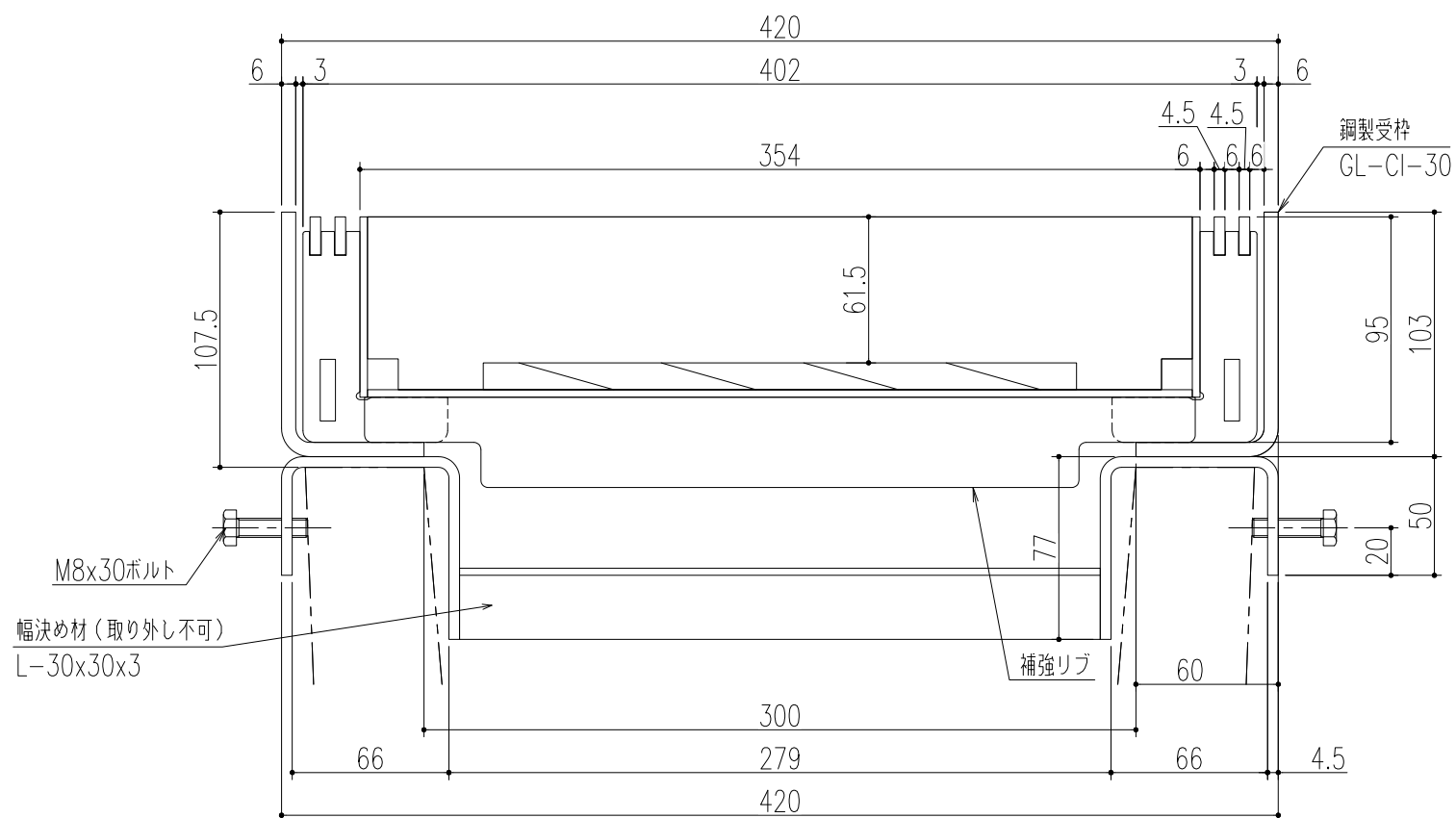
断面詳細図 S=1/3
