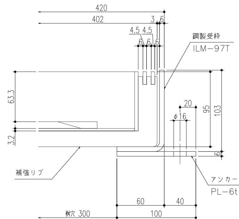
断面詳細図 S=1/3
