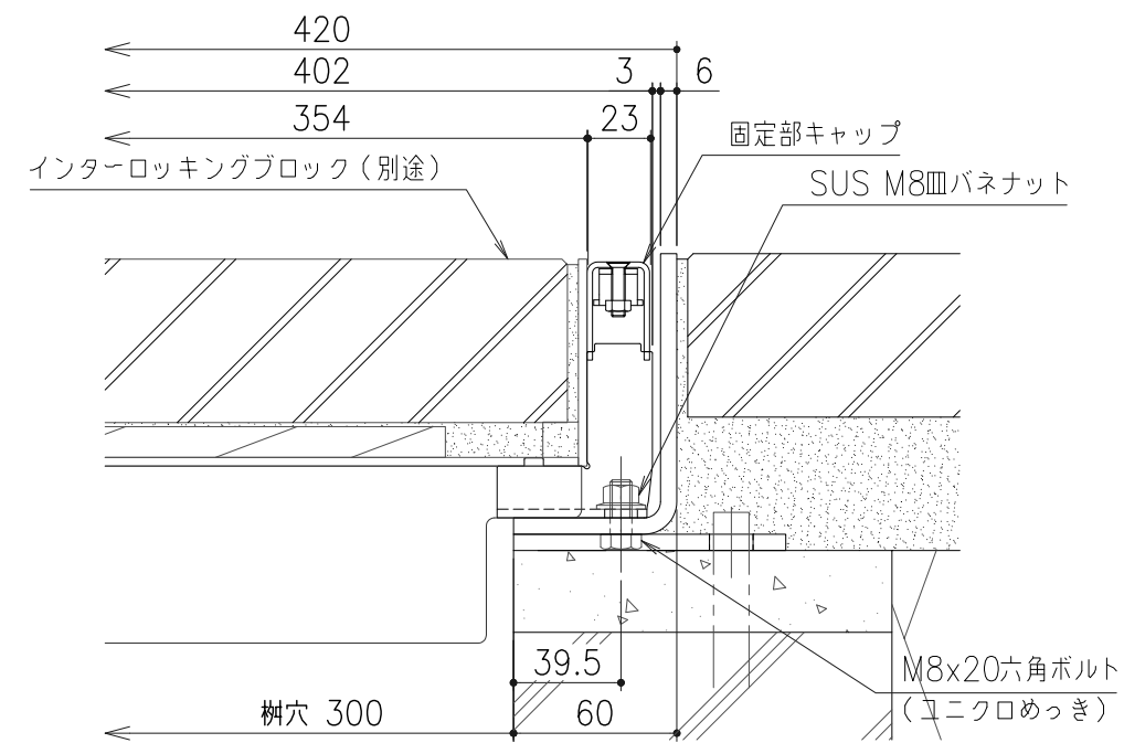
断面詳細図 (ボルト固定部) S=1/3
