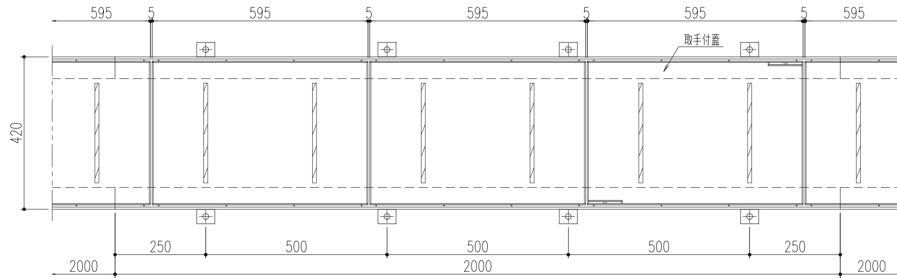
平面図 (S=1/10)
