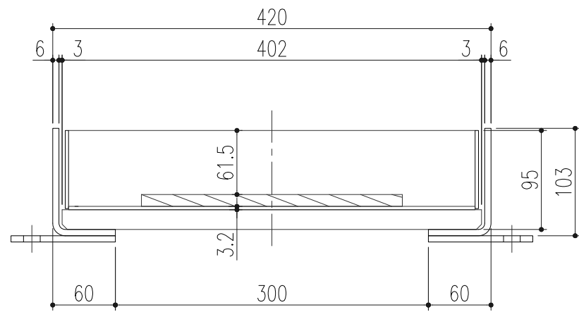
断面図 (S=1/5)
