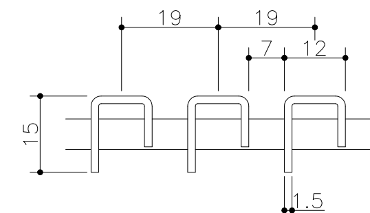
カバー断面詳細図
